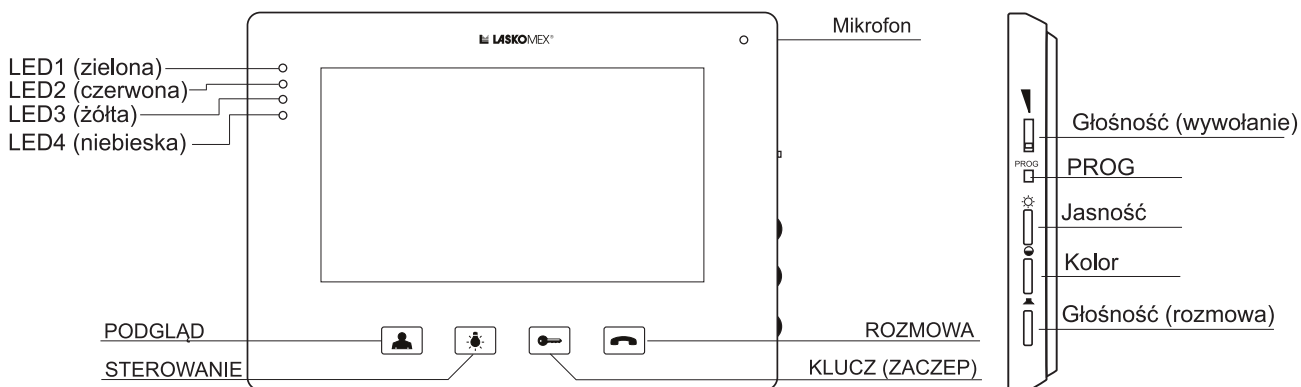
Rys. 1. Monitor MVC-8150
